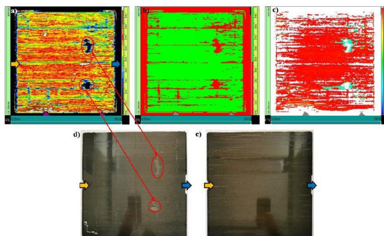
Figure 2 : Analyse par US de la santé matière des plaques composites carbone/vitrimère obtenues dans le cadre de l'étude a) Réponse en amplitude du signal US sur 12 couleurs, b) Réponse en amplitude du signal US sur 2 couleurs, c) Réponse en temps de vol du signal US, d) Face avant de la plaque composite analysée, e) Face arrière de la plaque composite analysée
