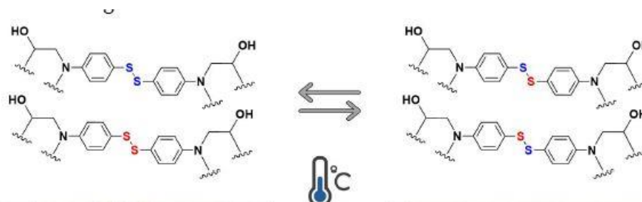
Figure 1 : Schéma de principe du réseau dynamique dans une résine époxy vitrimère avec le durcisseur de type 4-AFD.
