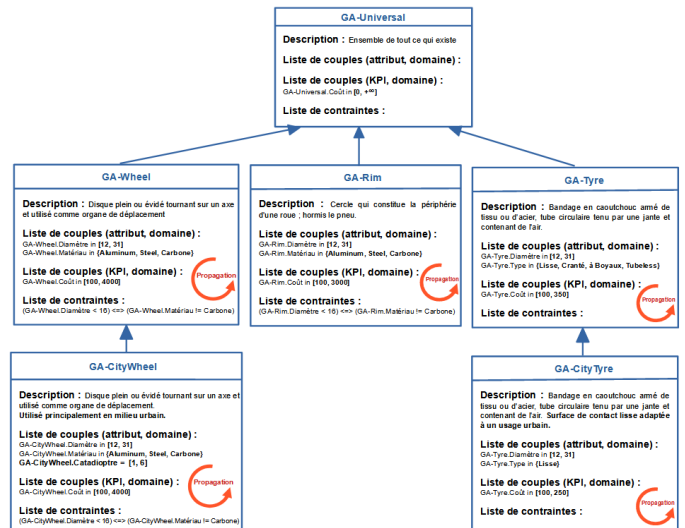
Fig. 3 : Ontologie de GA
