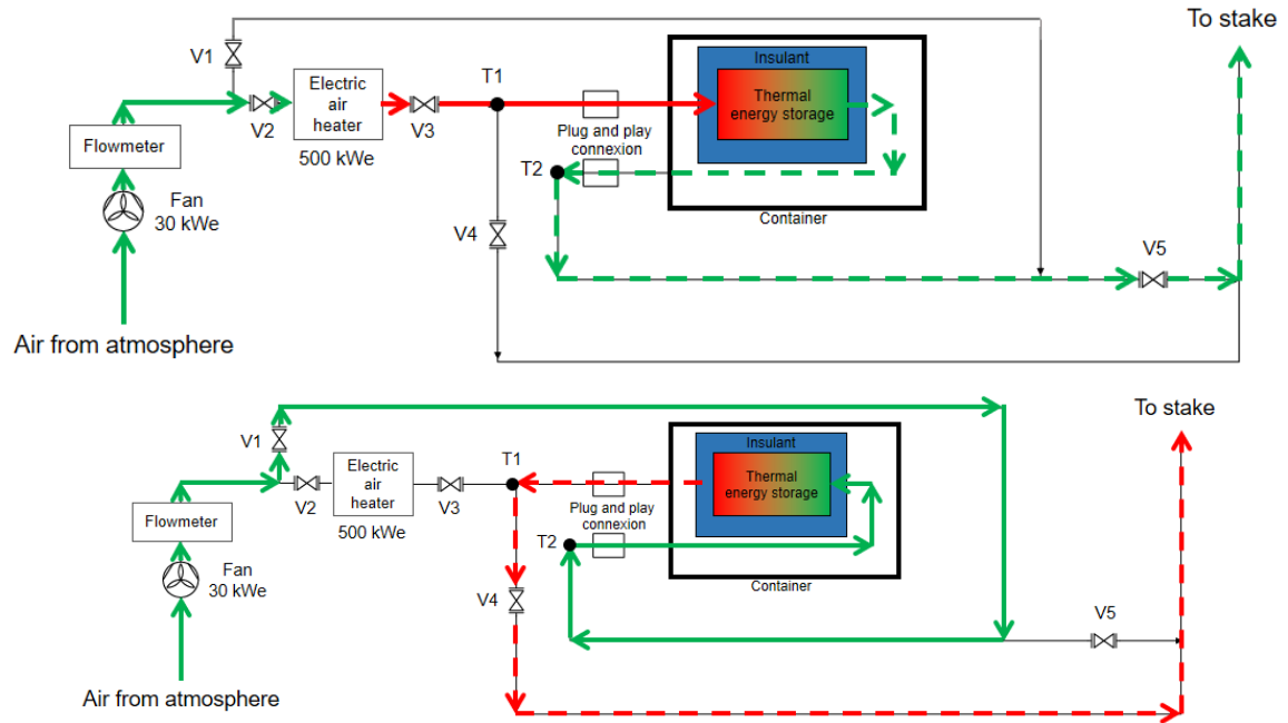
Figure 2: Schéma procédé banc de test durant la charge (en haut) et la décharge (en bas)
