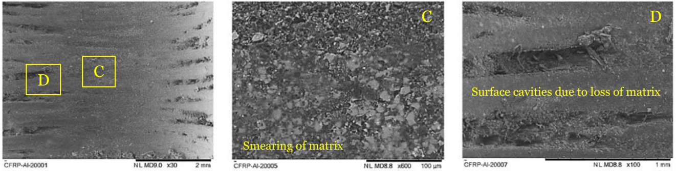
(b) CFRP/Al
